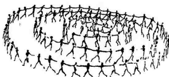
Universele cirkelbeweging
